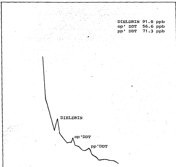
Figura 4. Cromatograma de la concentración de plaguicidas organoclorados totales en la estación 2 - de la laguna Carmen-Machona, Tabasco, México.
