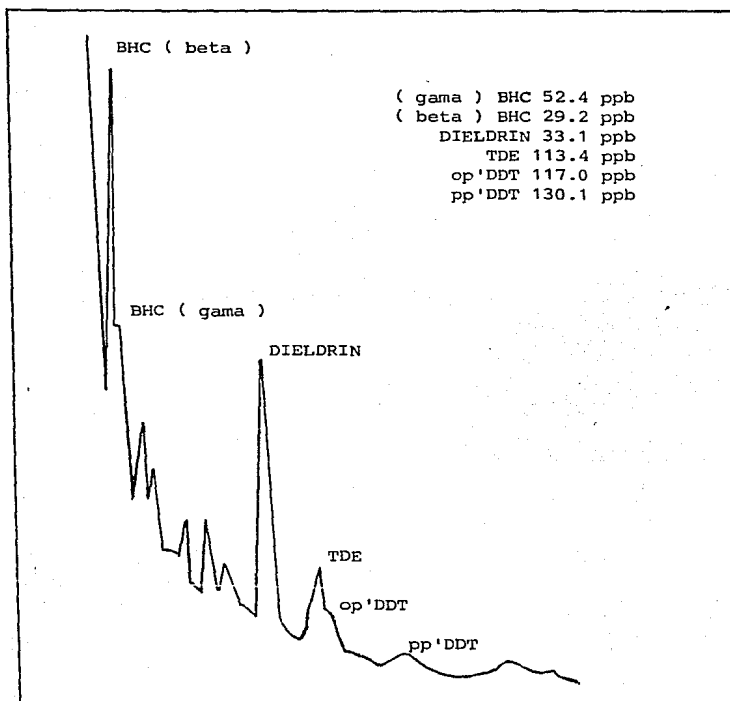
Figura 3. Cromatograma de la concentración de plaguicidas organoclorados totales en la estación 9 - de la laguna Mecocacán, Tabasco, México.
