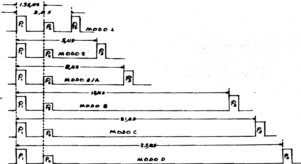
Fig. 3.5 Disposición de los pulsos en los modos de interrogación.
