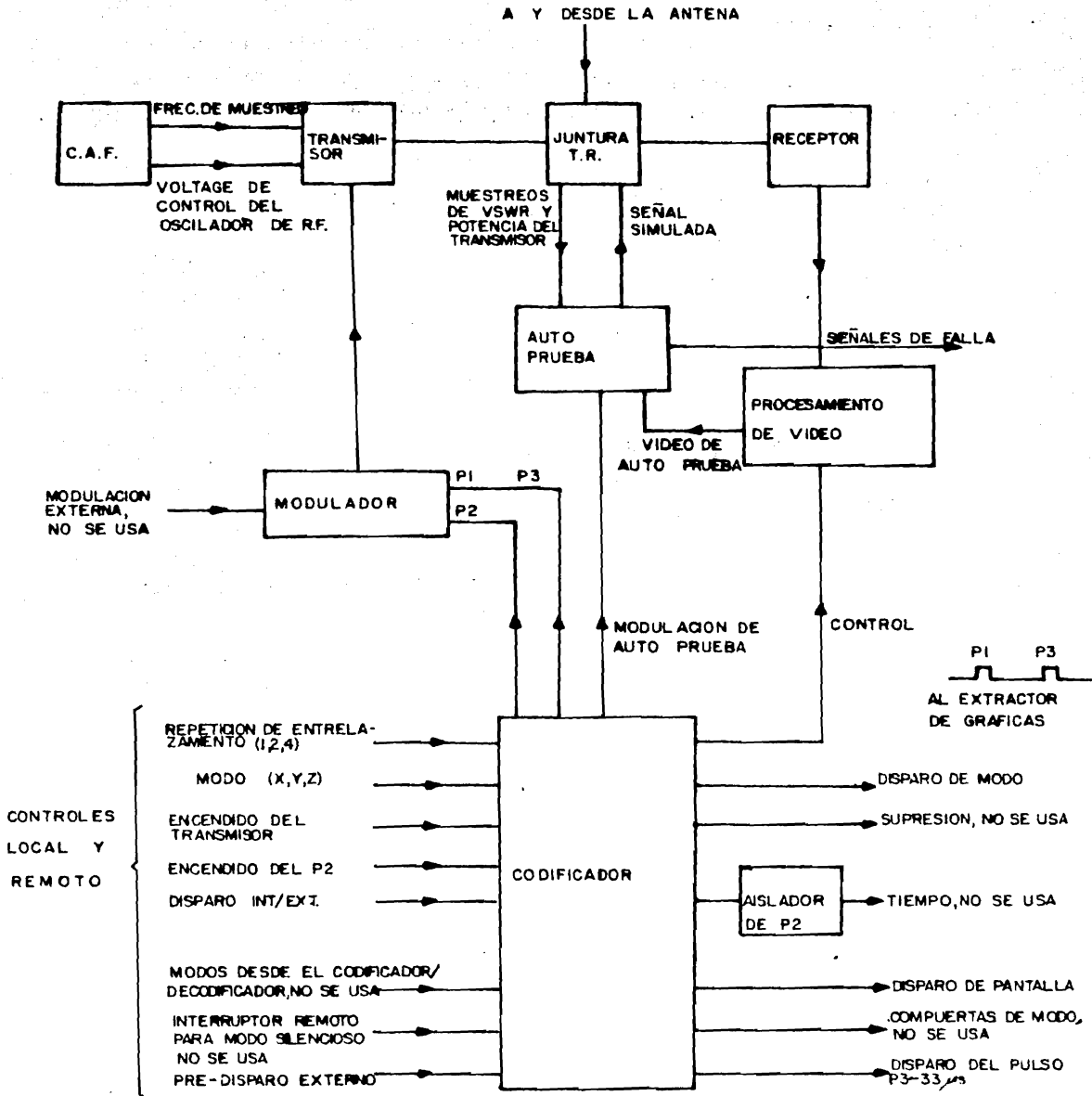
Fig. 4.1 Diagrama de bloques parcial del radar secundario.
