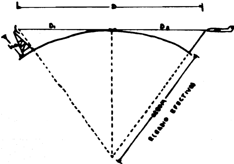
Fig. 2.16 Limitación de alcance por la curvatura de la tierra.
