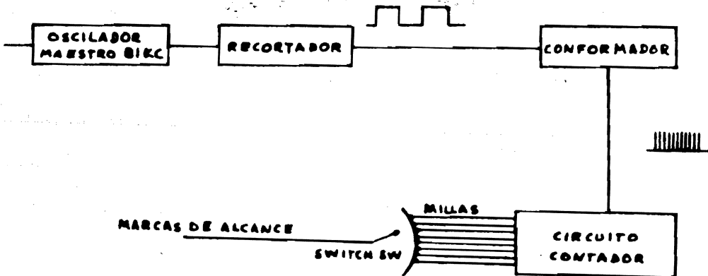
Fig. 2.8 Diagrama de bloques de un generador de marcas de distancia.
