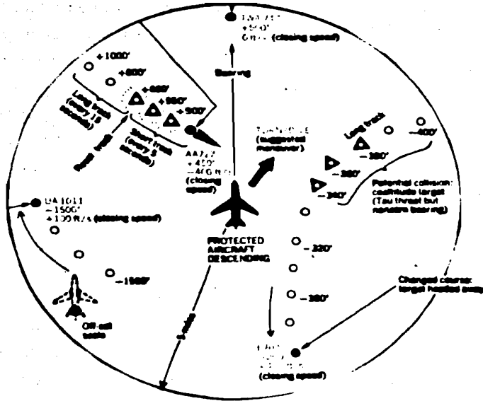
Fig. 5.32 BCAS Semiactivo de Litchford
