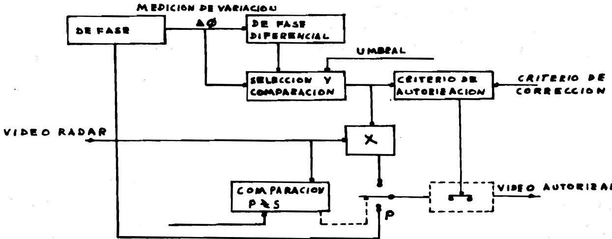
Fig. 2.11 Diagrama de bloques de un MTI.
