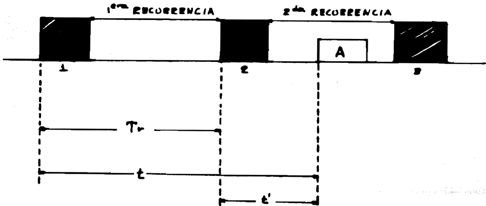
Fig. 2.17 Eco de Segunda recurrencia.
