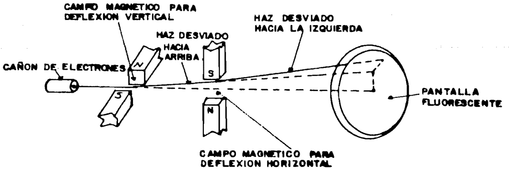
Fig. 2.5 Deflexión por campos magnéticos.
