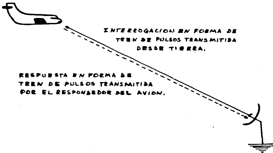
Fig. 3.2 Funcionamiento del radar secundario.
