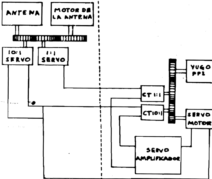
Fig. 2.10 Servomecanismo de conexión antena-bobinas.
