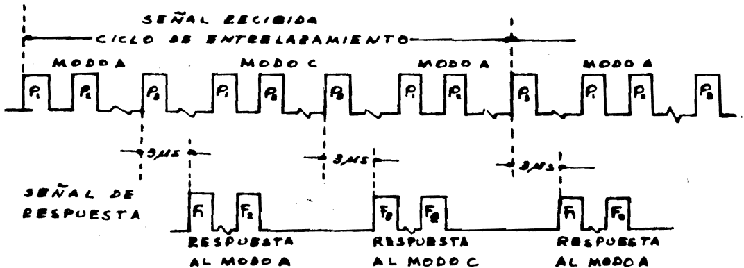
Fig. 3.7 Señales recibidas y transmitidas por el respondedor.
