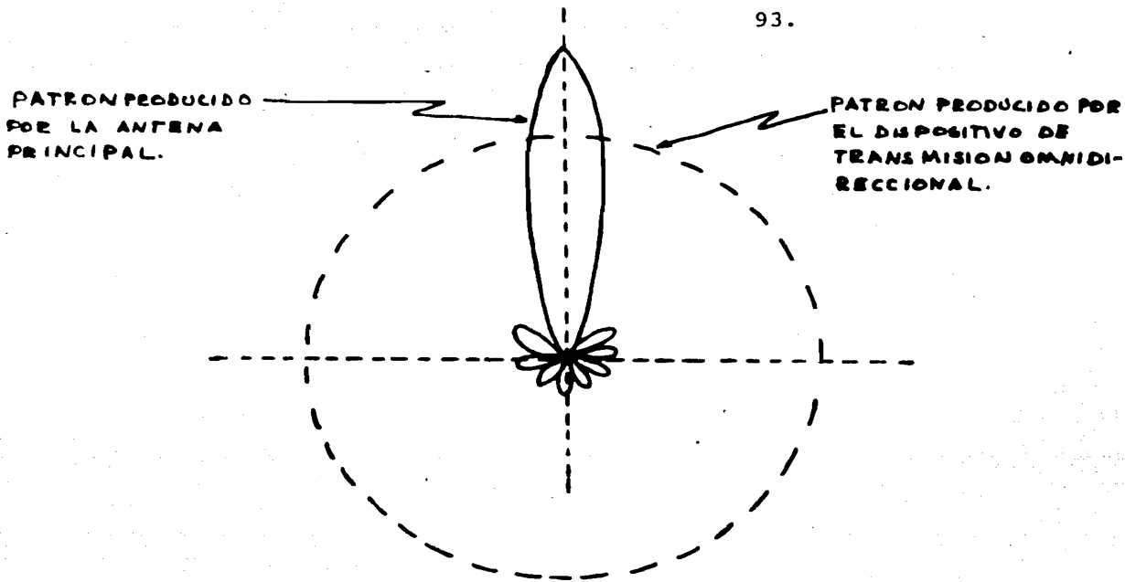
Fig. 3.12 Patrón de radiación horizontal para un sistema de SLL usando un dispositivo de transmisión omnidireccional.
