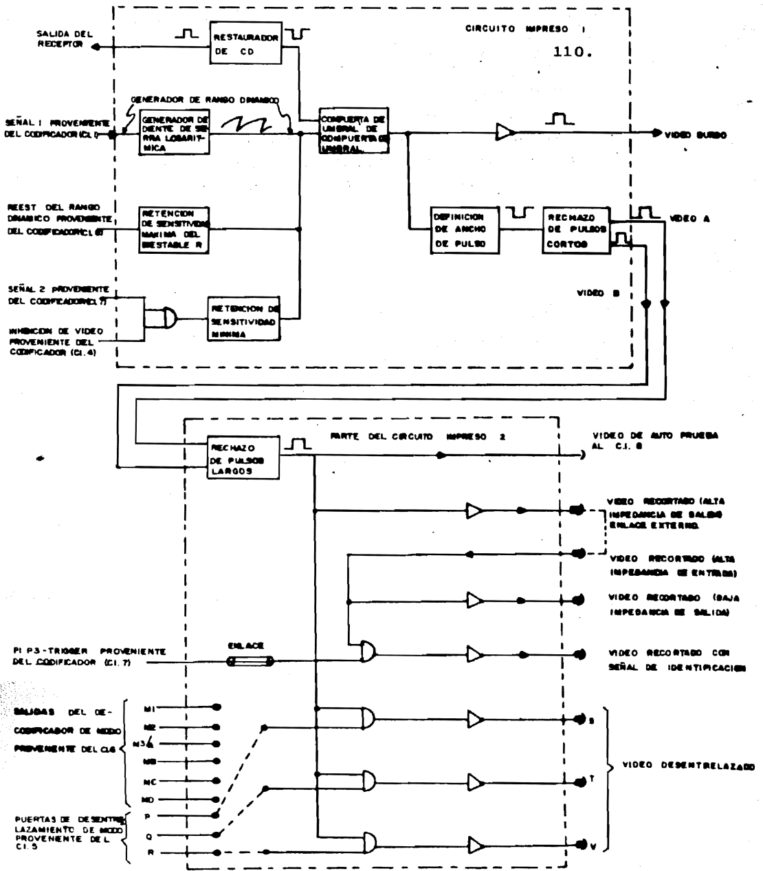
Fig. 4.3 Diagrama de bloques para procesamiento de video.
