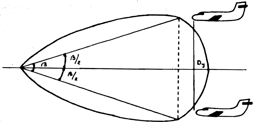
Fig. 2.18 Resolución angular.
