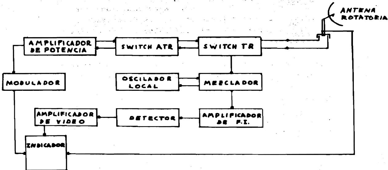
Fig. 2.1 Diagrama de bloques de un sistema típico de radar.
