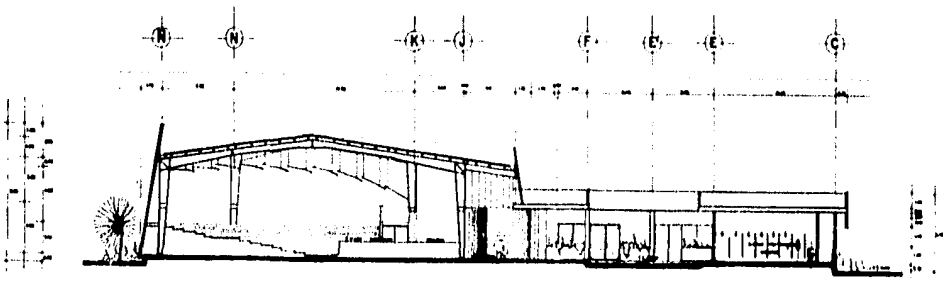
CORTE SECCION 2-2
