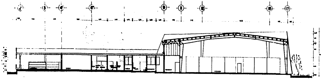
CORTE SECCION 1-1
