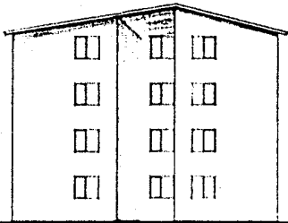
FACHADA LATERAL esc. 1/75
