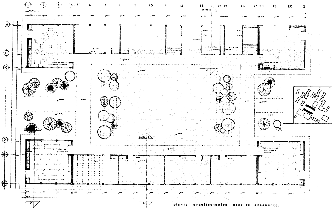
planta arquitectonica area de enseñanza.
