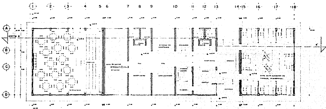
planta arquitectónica, administración y biblioteca.
