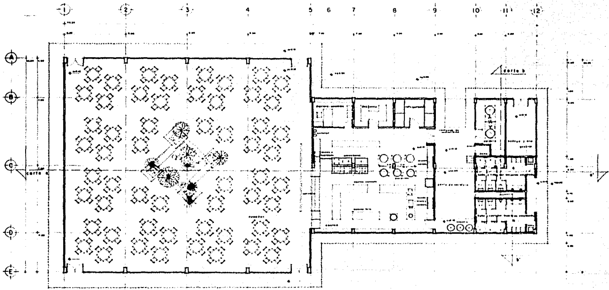
planta arquitectonica, comedor, cocina y servicios. 000 1-79.
