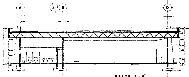
corte A-A. esc. 1:75
