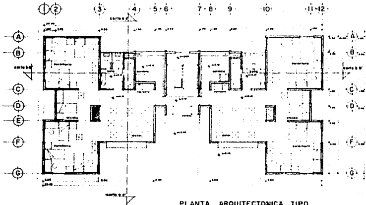
PLANTA ARQUITECTONICA TÍPO vivienda niños esc. 1/75 (planta baja, 3 niveles).
