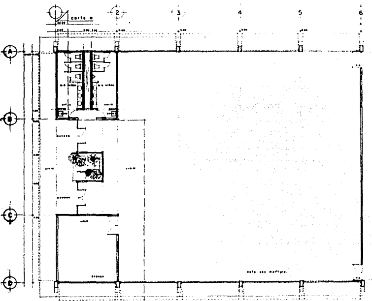
planta arq. aula de usos múltiples. esc. 1:75
