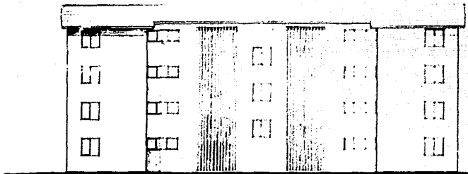
fachada posterior. esc. 1/75
