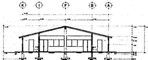
corte b-b. esc. 1/75
