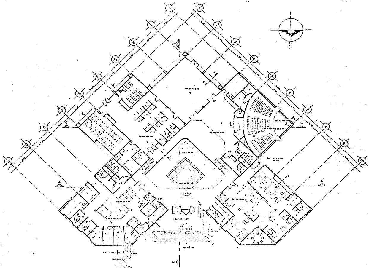
PLANTA BAJA
