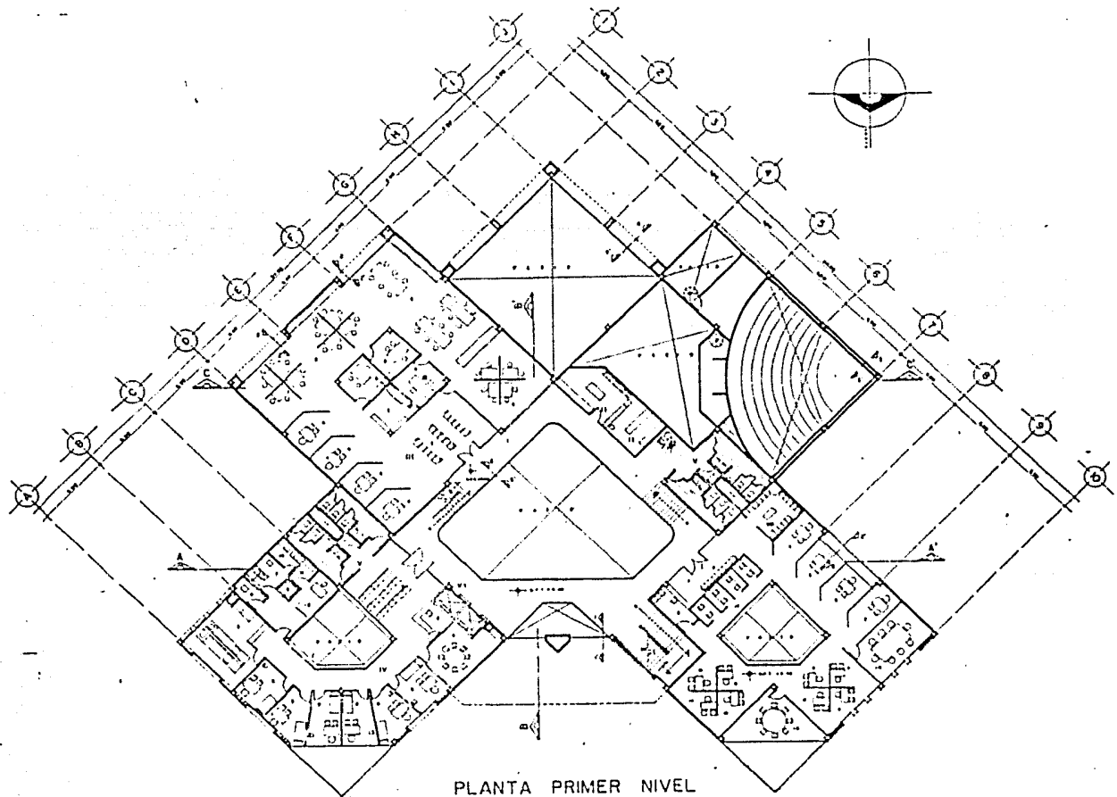
PLANTA PRIMER NIVEL
