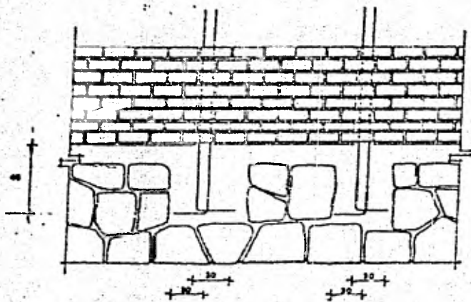
ANCLAJE DE CASTILLOS
