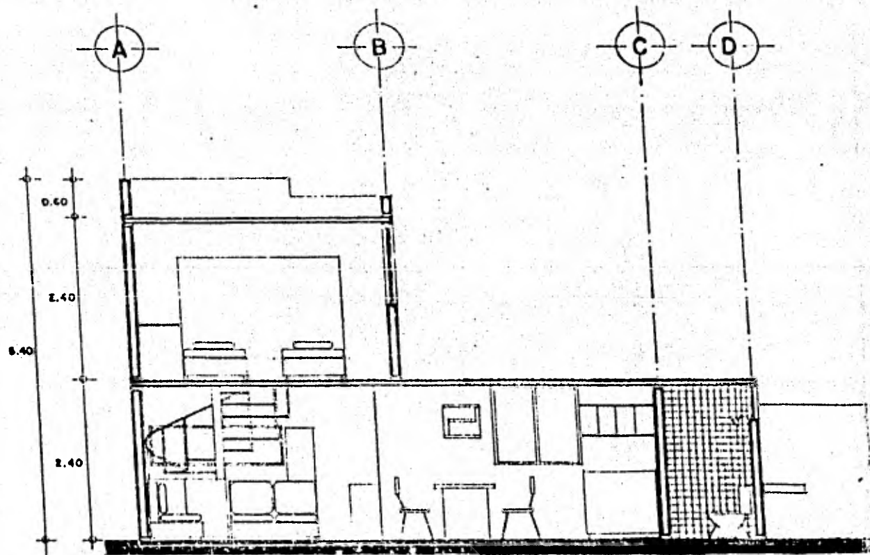
CORTE LONGITUDINAL
