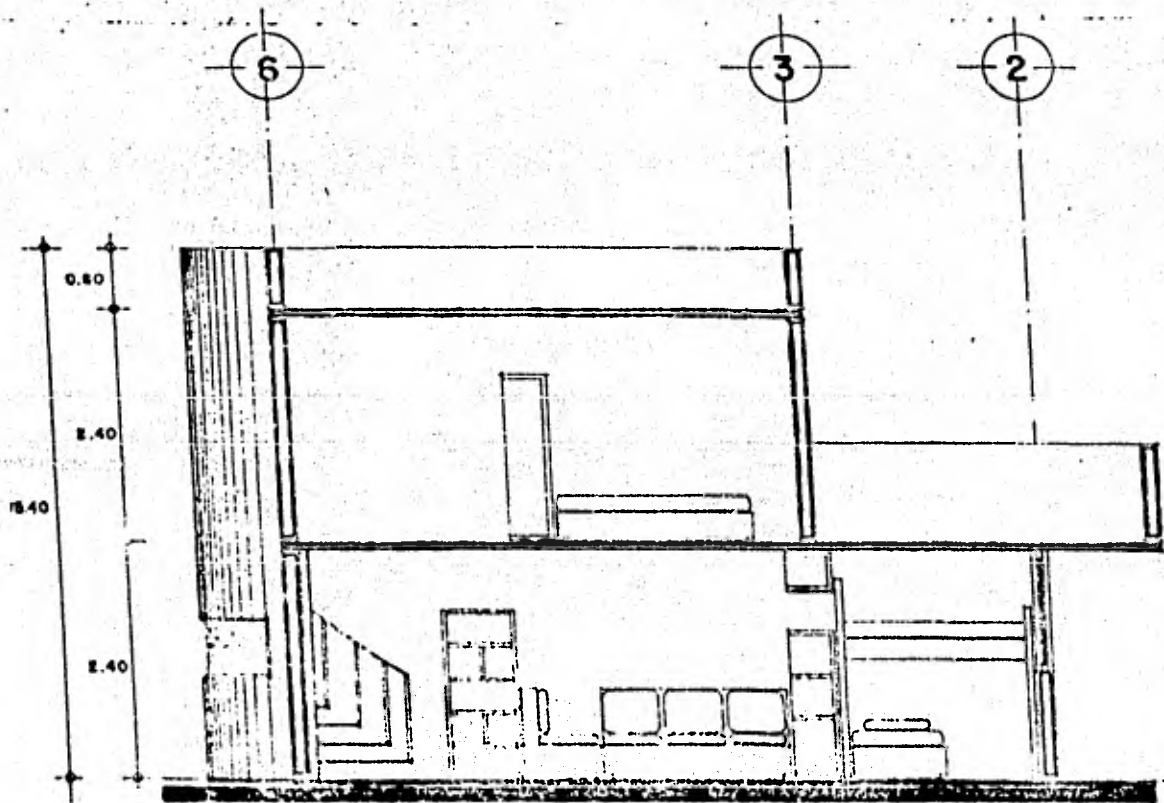
CORTE TRANSVERSAL
