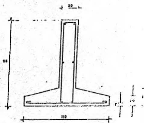
CORTES DE CIMIENTOS
