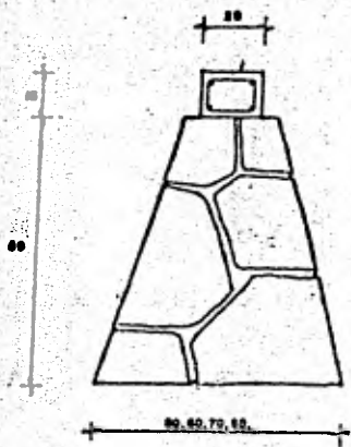
CORTES DE CIMIENTOS
