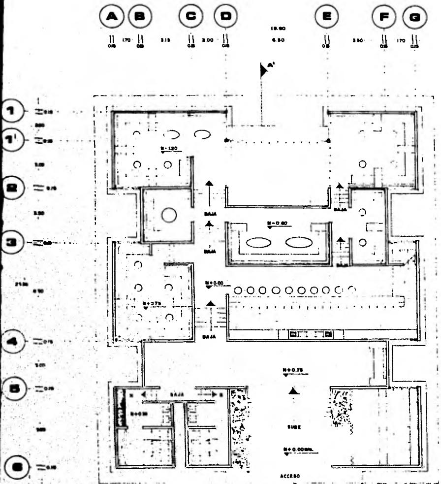
PLANTA DISCOTEQUE
