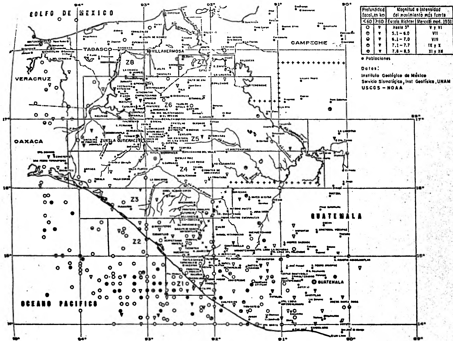
Fig 1. Carta sísmica del estado de Chiapas
